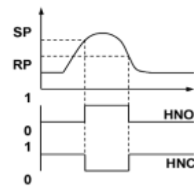
Fig.: Hysteresis function
